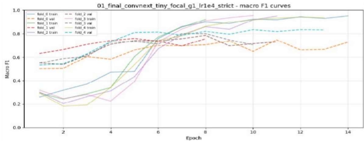
Figure 5.4: ConvNeXt-Tiny macro F1 curves
