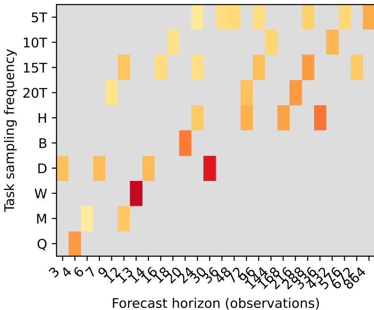
chronos2
