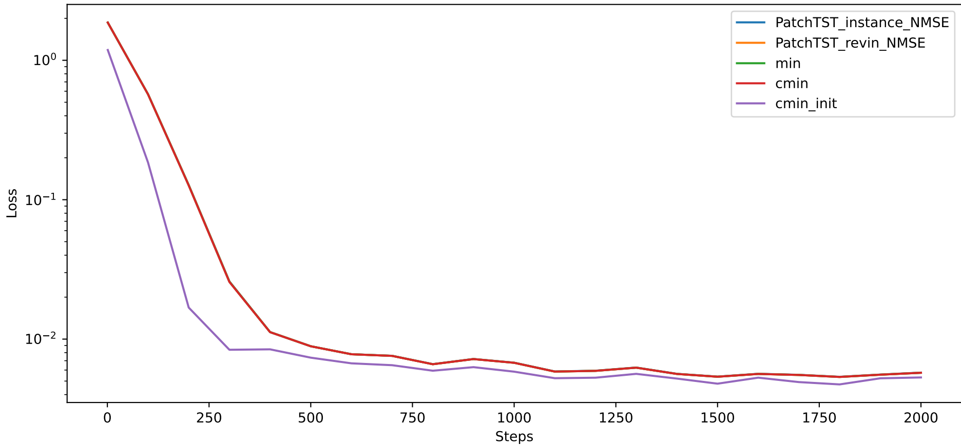
Valid2 NMSE
