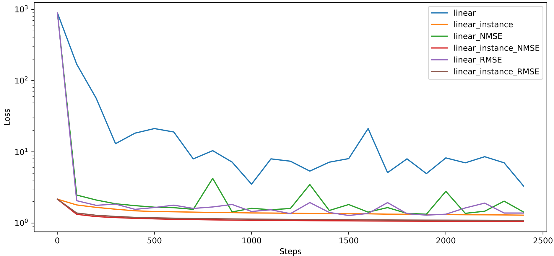
Valid2 NMSE
