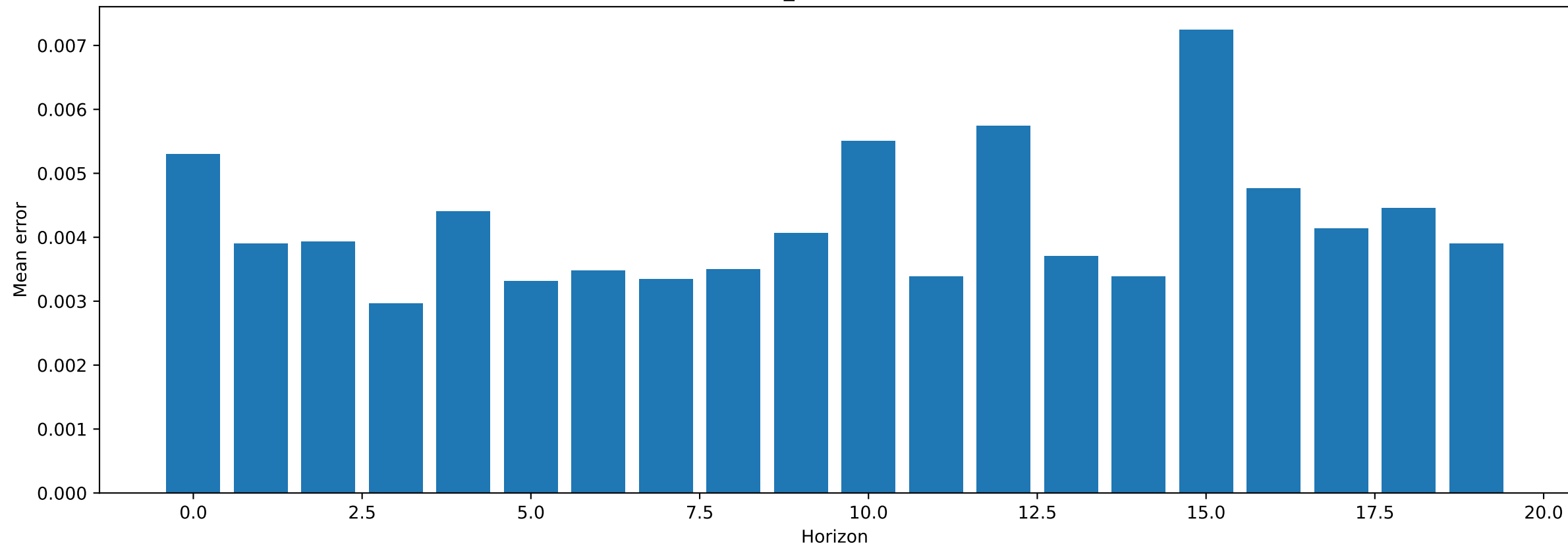
Test 1 MSE of PatchTST_revin : 0.004223770461976528
