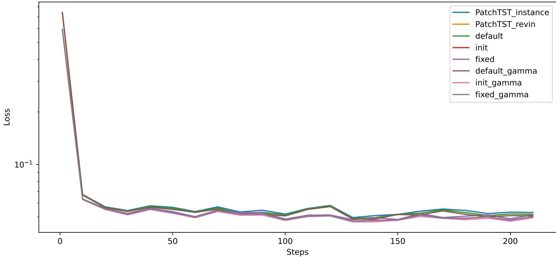
Valid MAE
