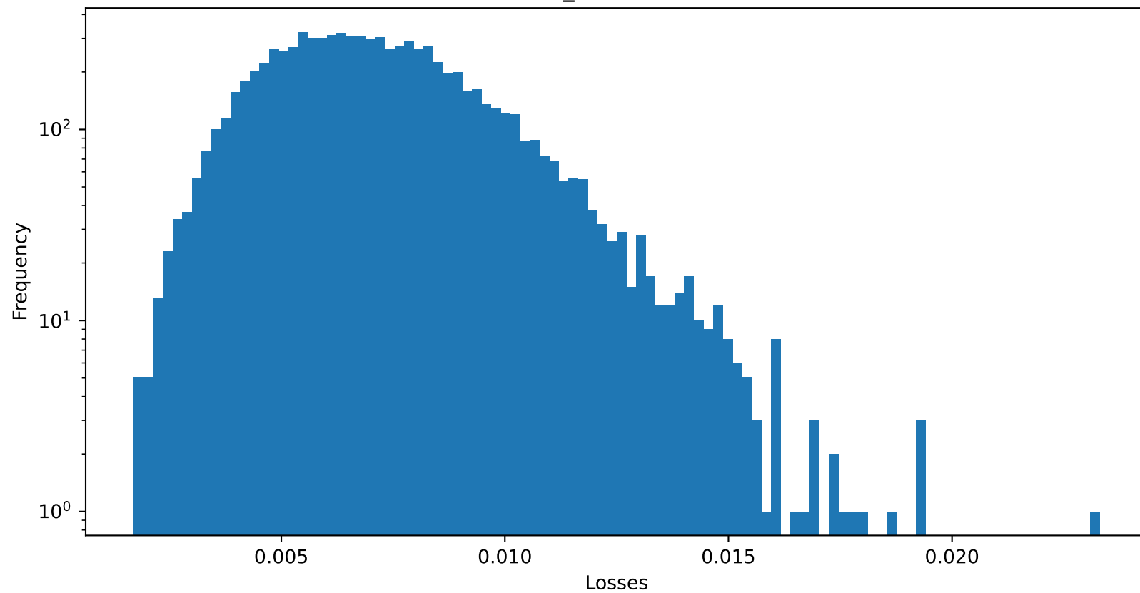
Test 2 NMSE of PatchTST_revin : 0.0071537490002810955
