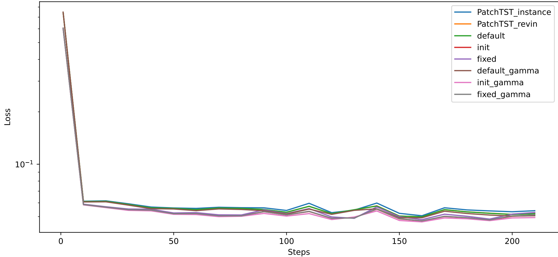
Valid3 MAE
