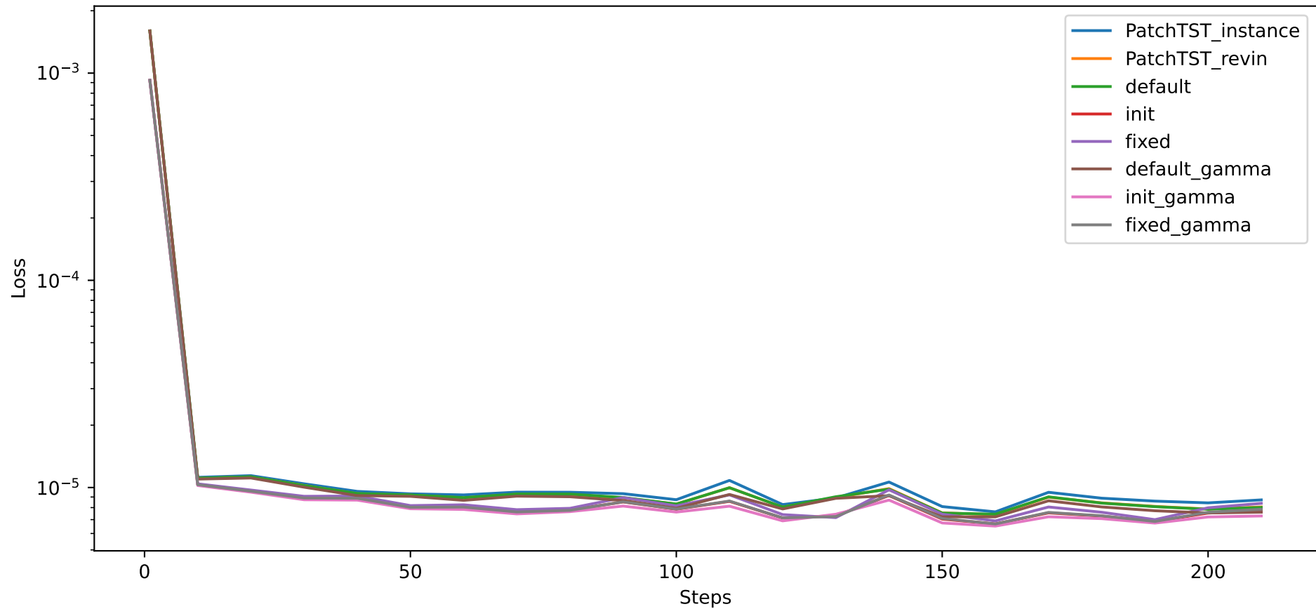
Valid RMSE
