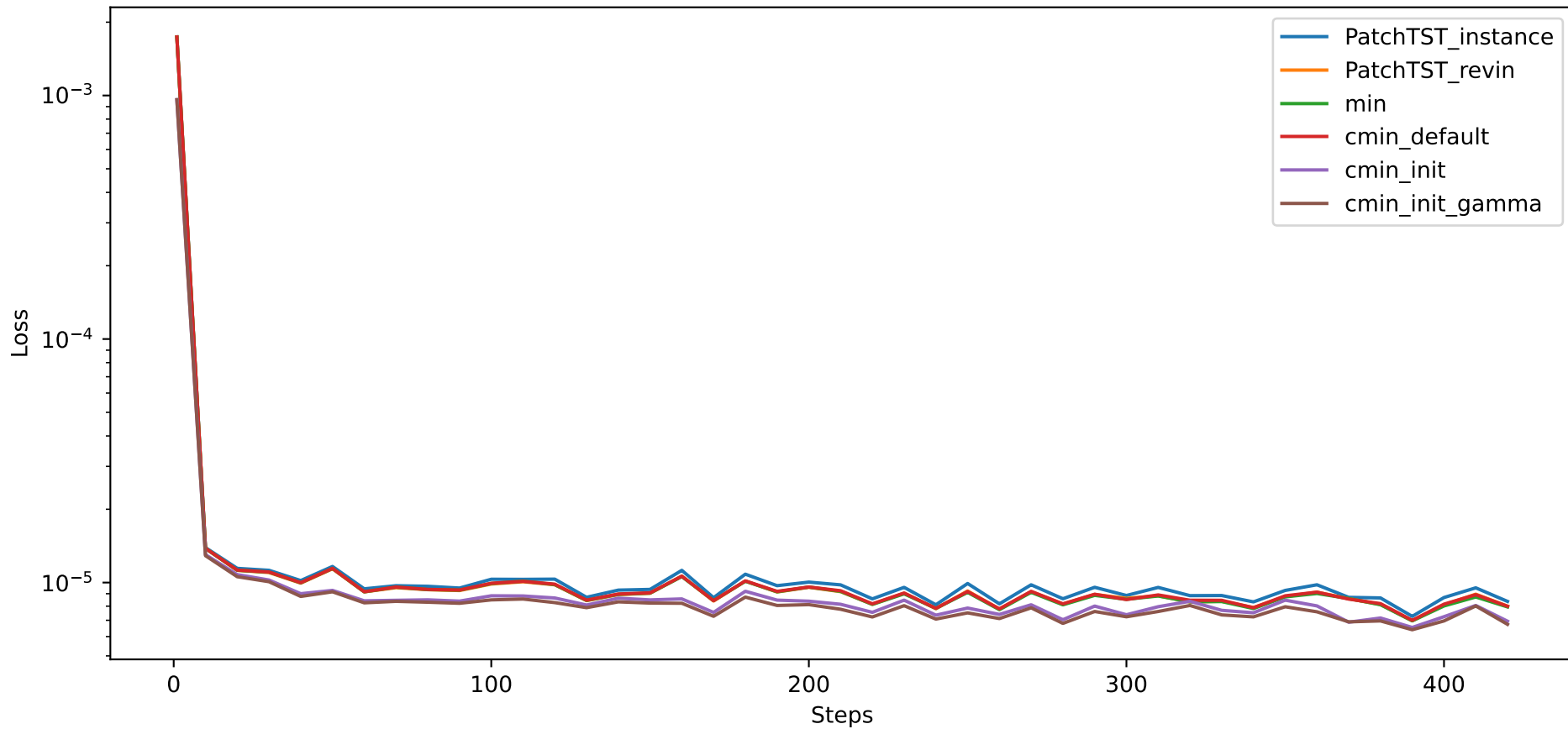
Valid2 RMSE
