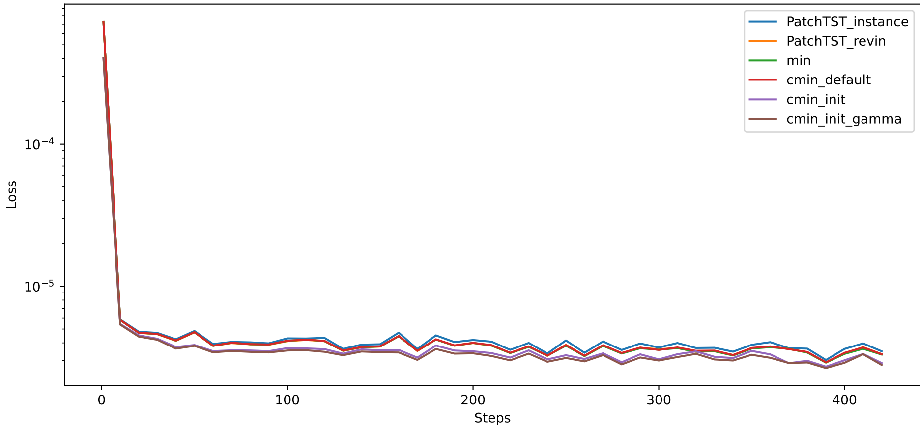
Valid3 RMSE
