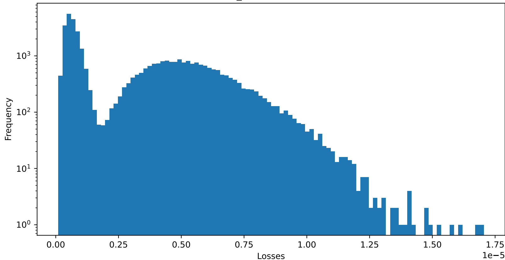
Test 1 RMSE of PatchTST_instance : 3.0920687095203903e-06
