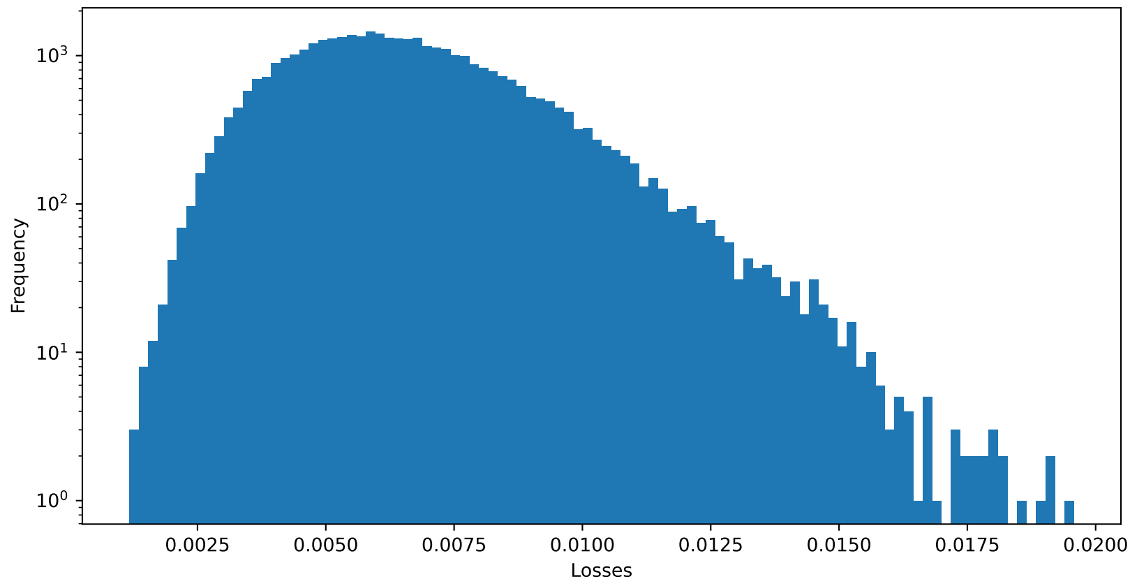
Test 1 NMSE of min : 0.006570378318428993
