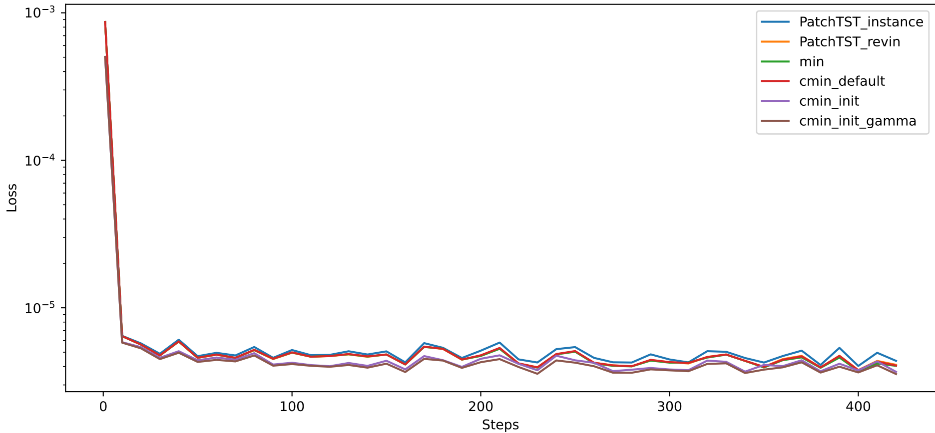
Valid RMSE
