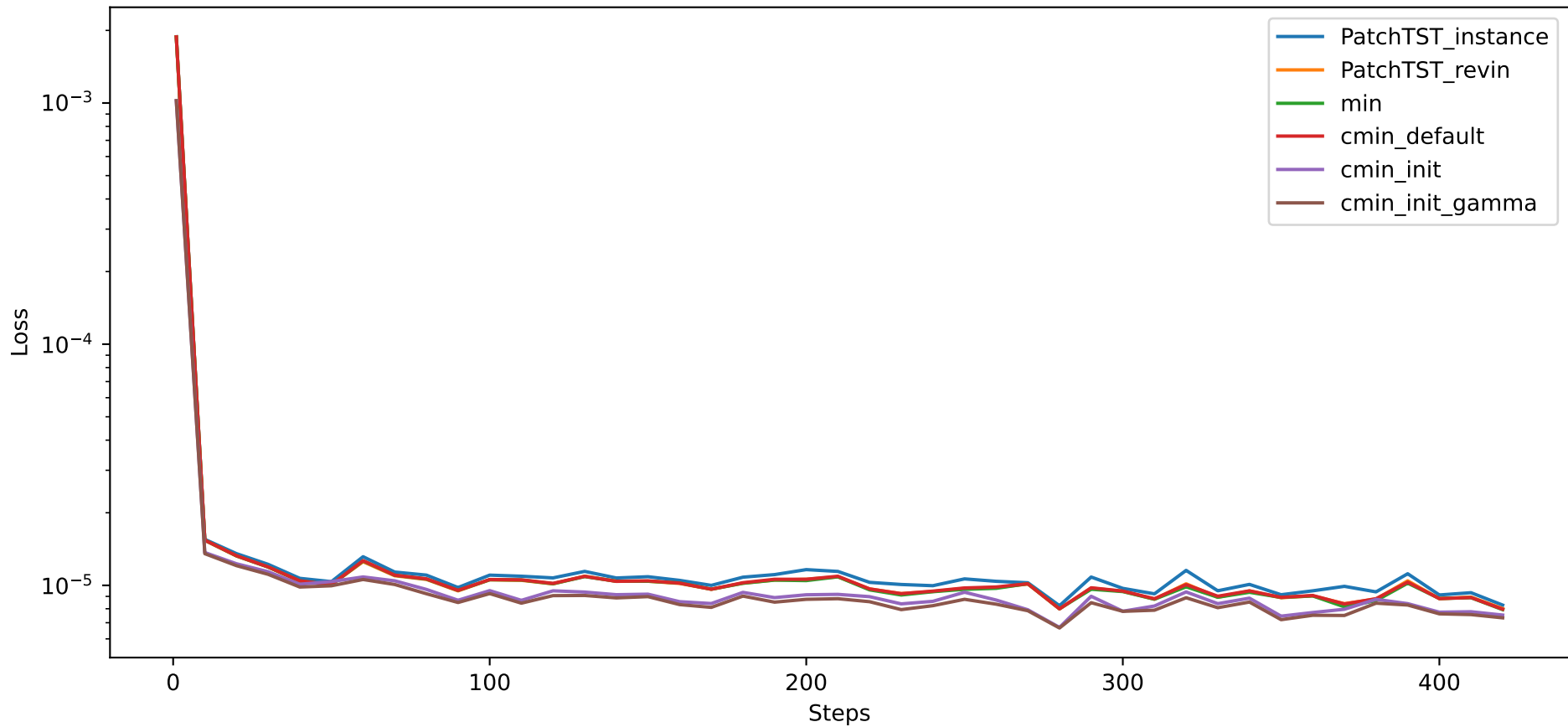
Valid2 RMSE
