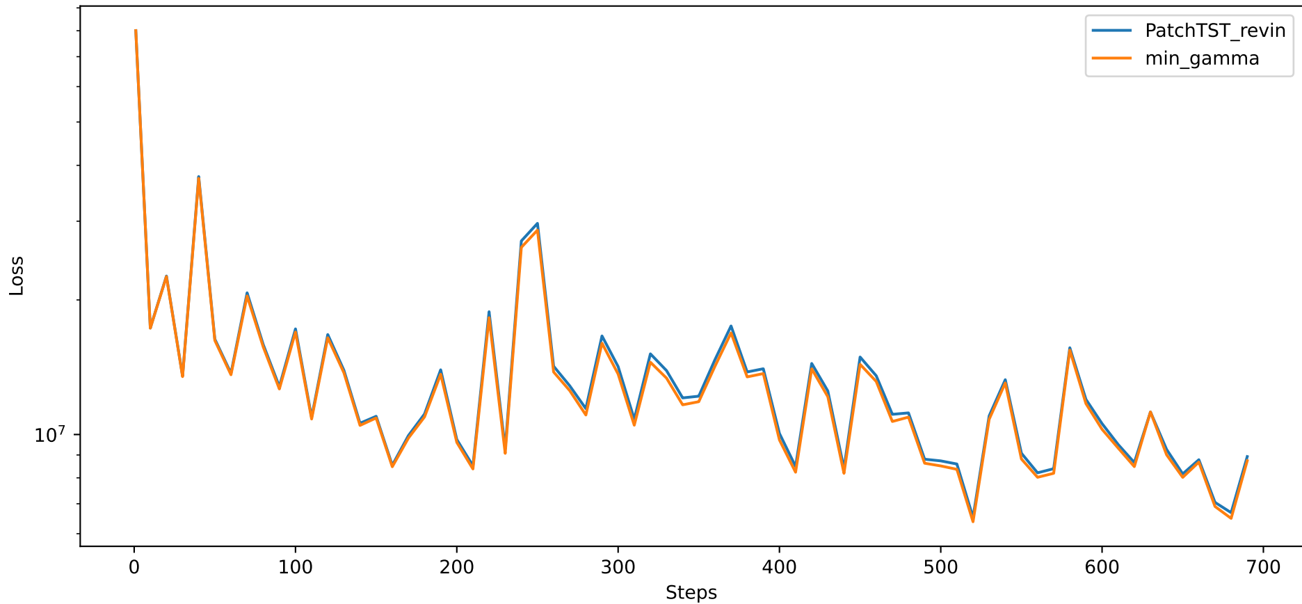
Valid MSE
