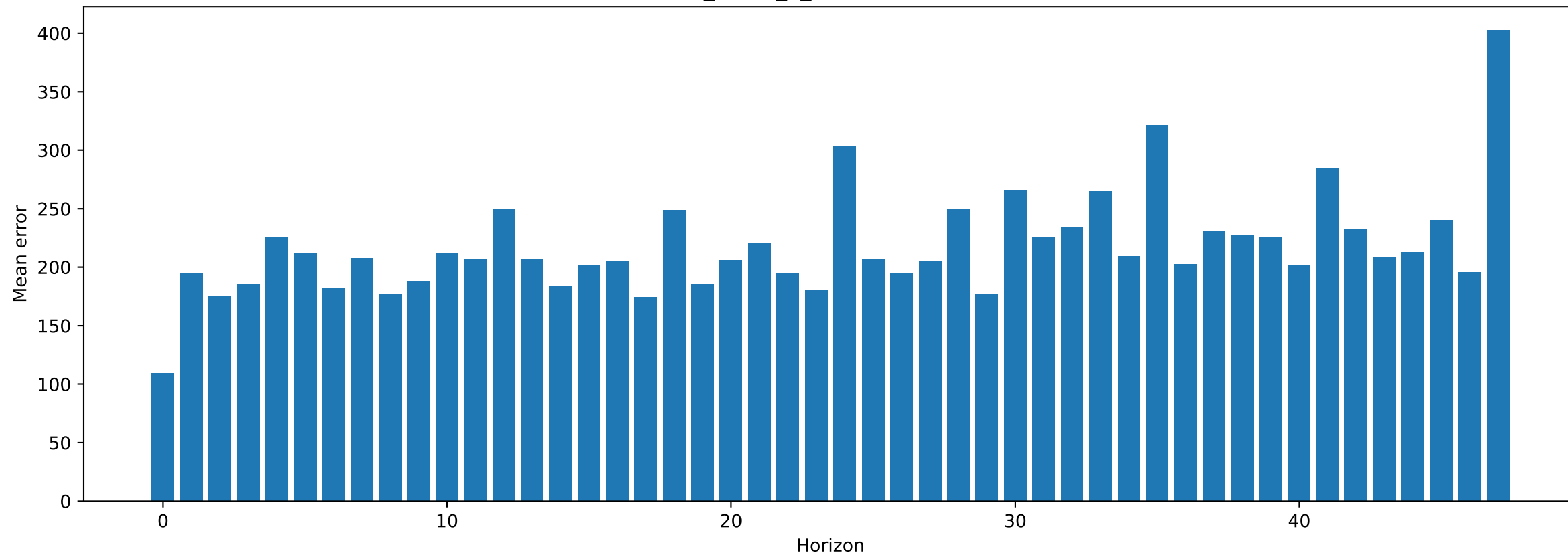
Test 2 MAE of PatchTST_NMSE_2_removeFalse : 217.88088989257812
