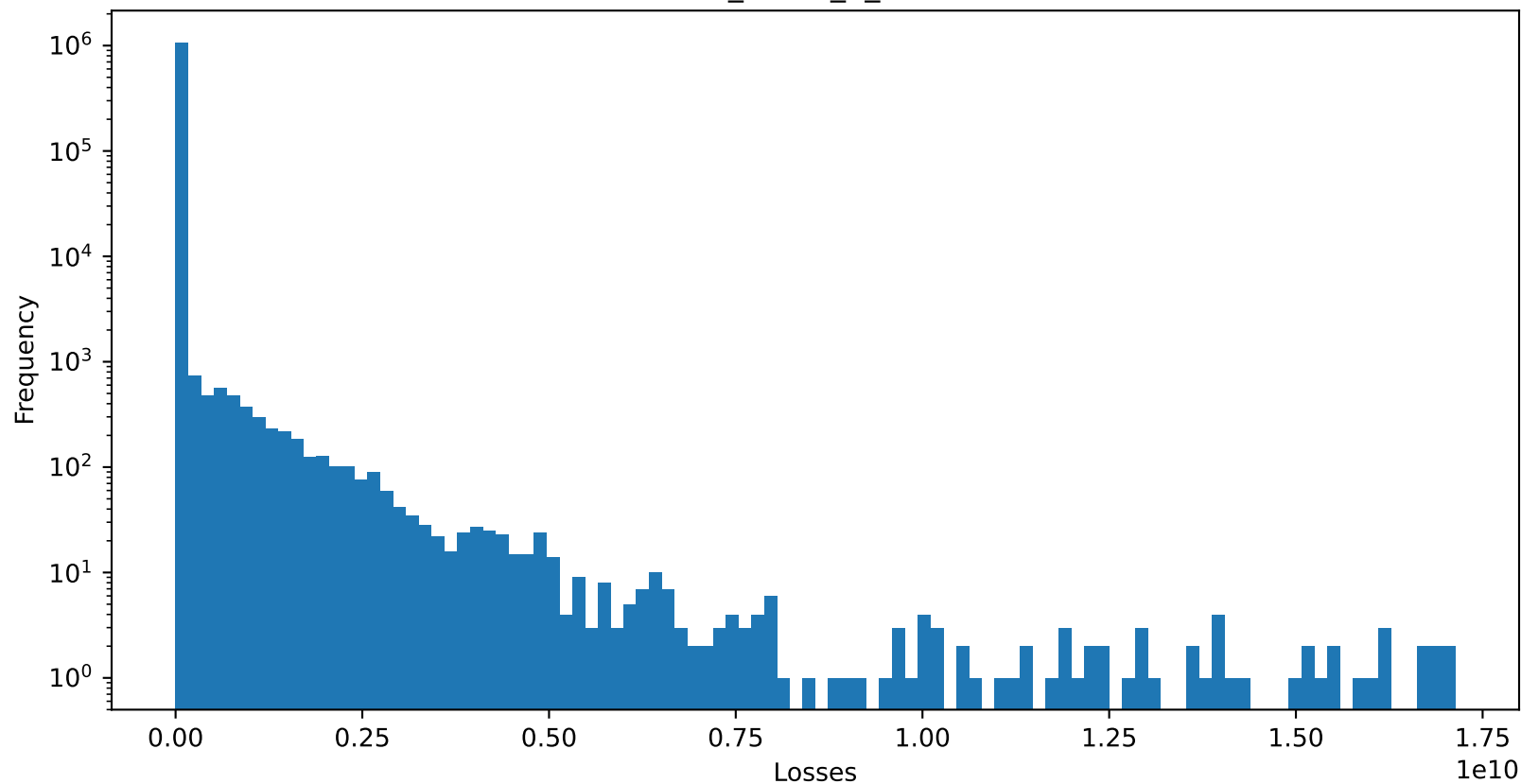
Test 1 MSE of PatchTST_NMSE_2_removeTrue : 6732824.5
