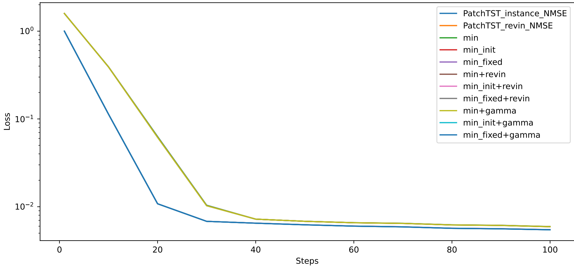
Valid3 NMSE
