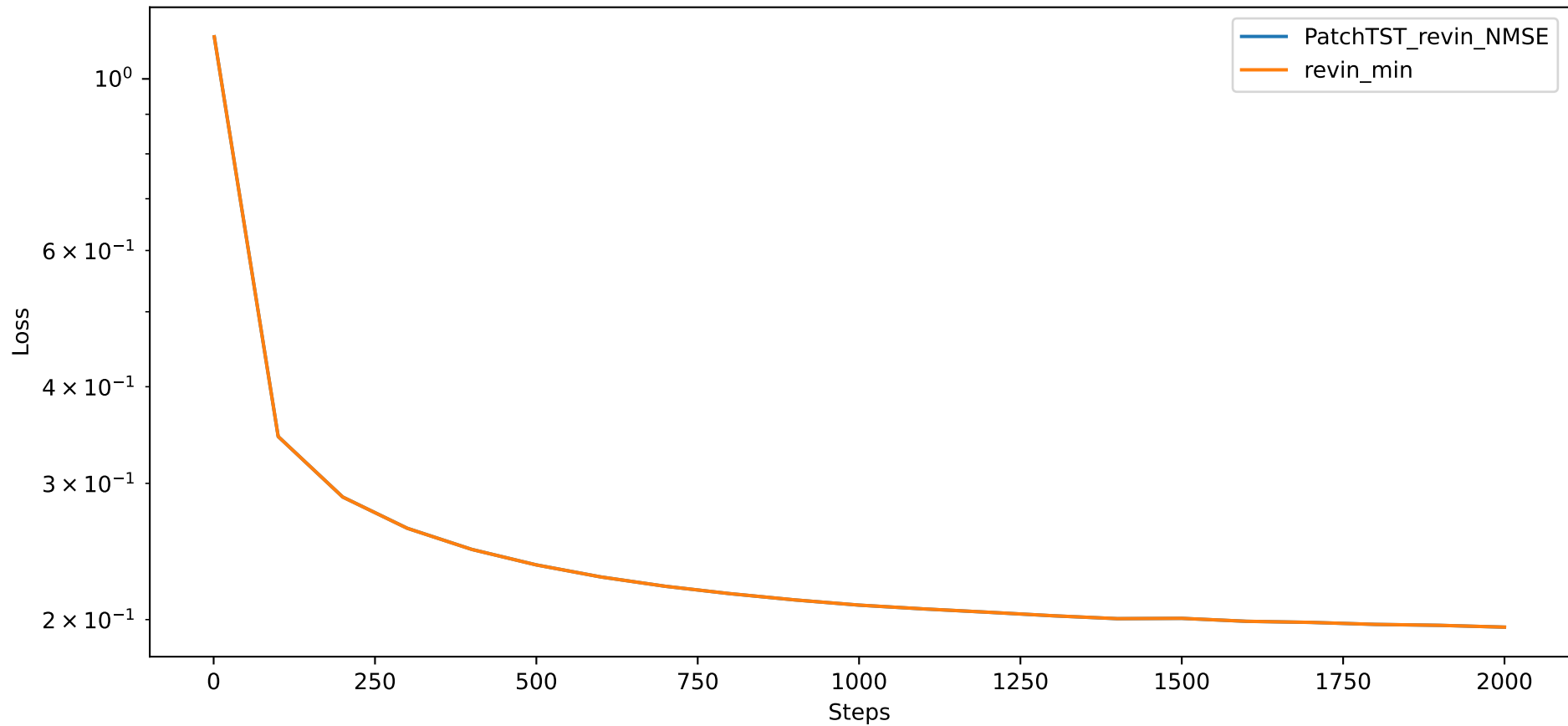
Valid3 NMSE
