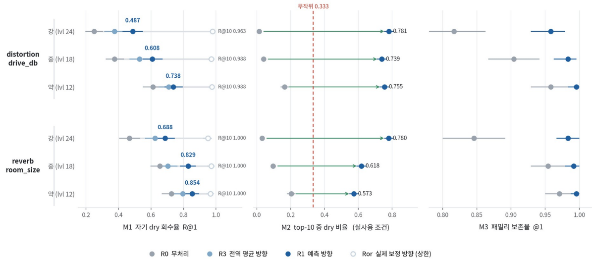
그림 7. Q6 — 검색 경로. M1 자기 dry 회수율, M2 실사용 조건의 dry 비율, M3 패밀리 보존율. 세 조건이 모두 충족되어야 성공으로 판정한다.
