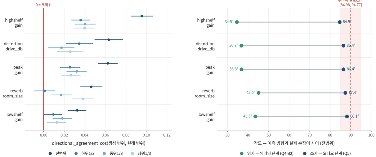
그림 6. Q5 — 생성 경로의 directional_agreement(왼쪽)와 읽기·쓰기 각도 대조(오른쪽). 붉은 띠는 무작위 널의 95% 범위이다.
