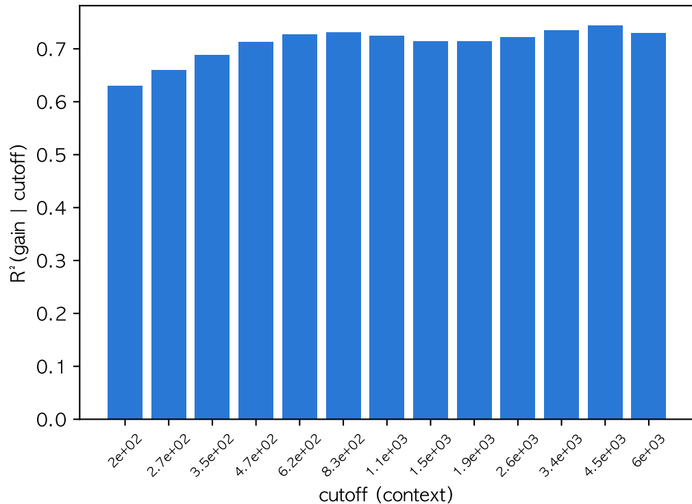
context별 held-out R^2 (회색=검정력 부족)
