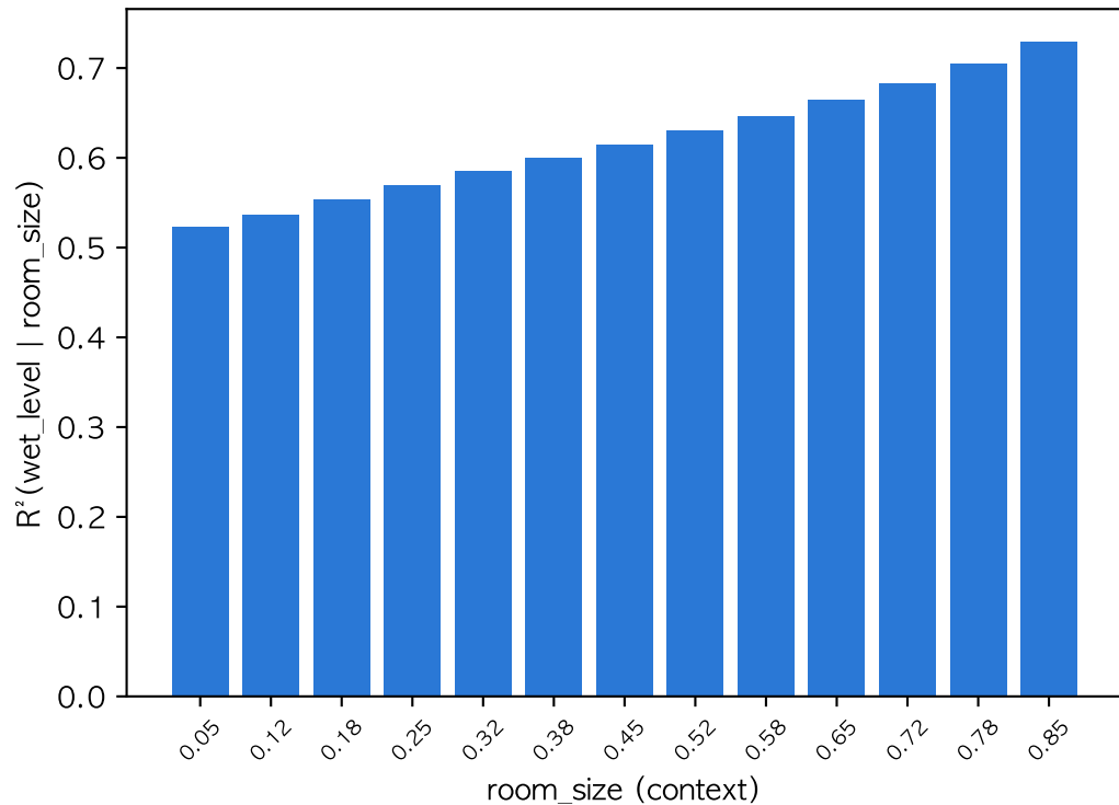
context별 held-out R^2 (회색=검정력 부족)
