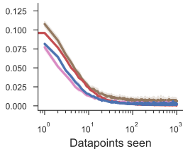
Sinusoid regression
