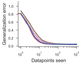
Linear regression
