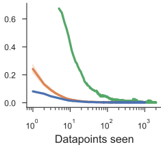
Sinusoid regression
