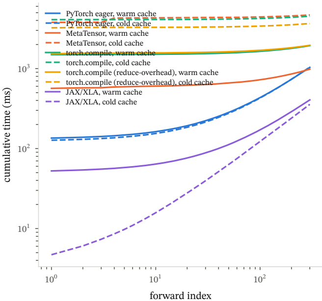
distilgpt2
