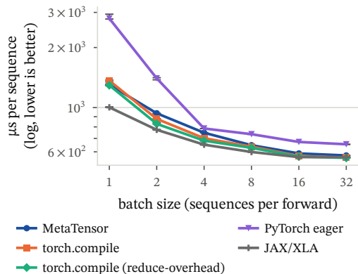
distilgpt2
