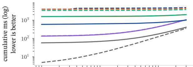
gpt2
