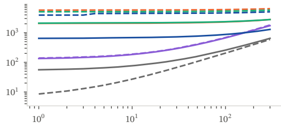
gpt2
