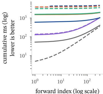
distilgpt2
