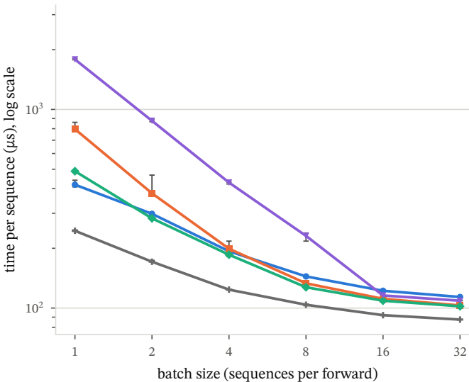
bert-mini
