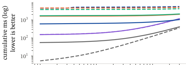
gpt2
