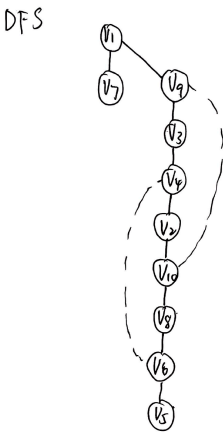
图 2 从 v_1 开始的深度优先搜索树
