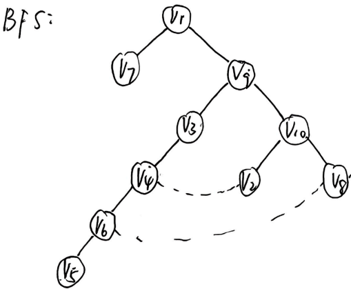
图 1 从 v_1 开始的广度优先搜索树
