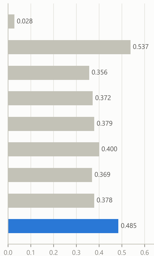
Macro-F1
