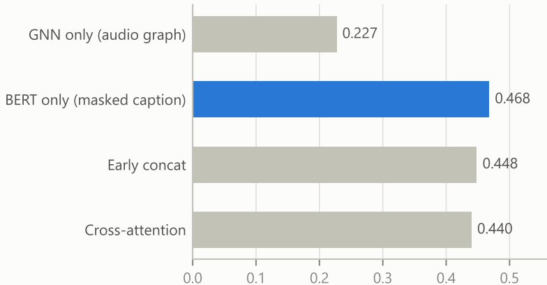
Macro-F1
