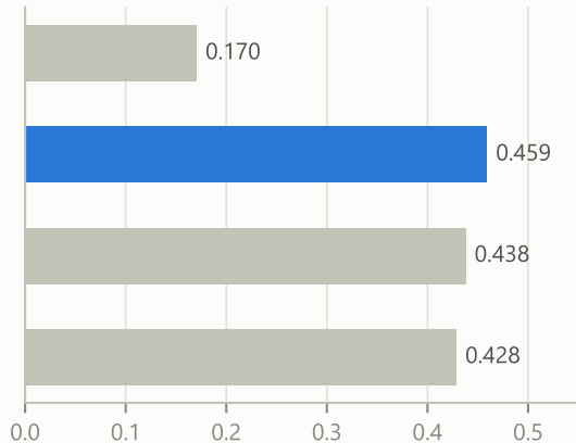
AUC-PR
