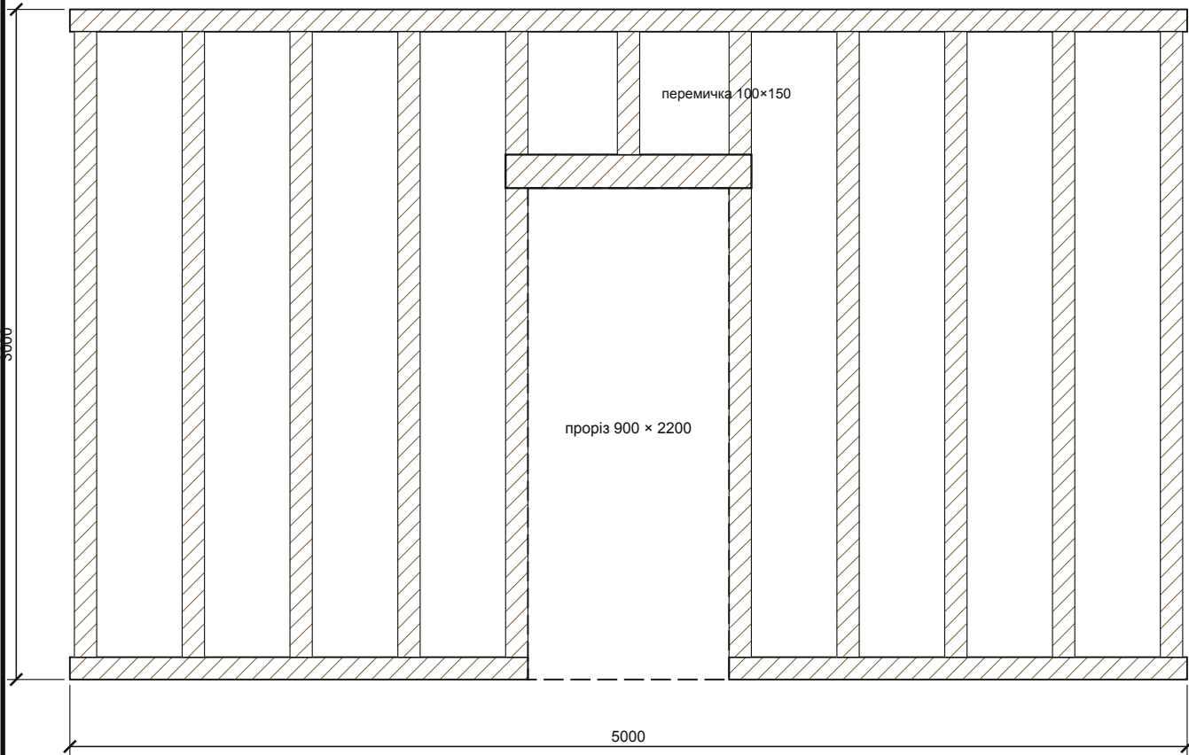
Каркас південної стіни, М 1:30
