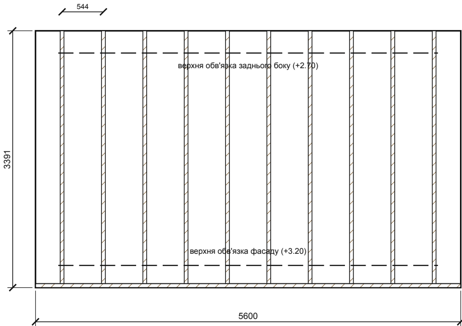
План крокв, М 1:50
