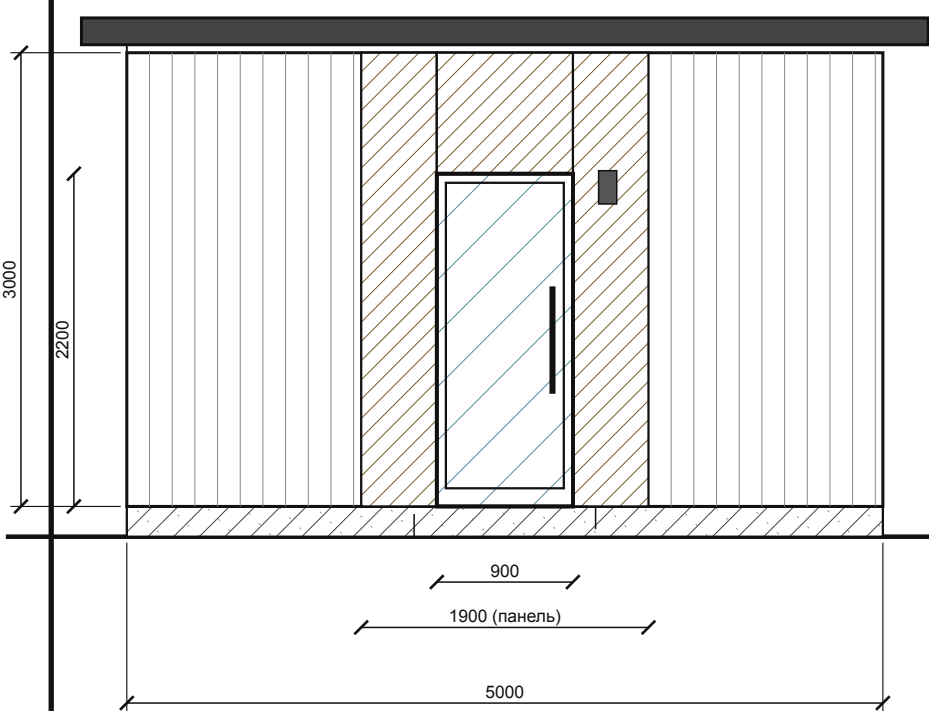
Фасад 1–5 (південний, вхід)
