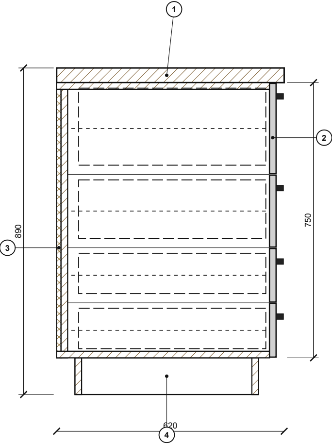
Переріз шафи №2, 1:10
