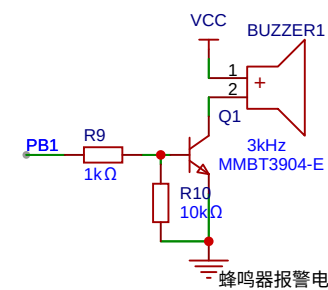
蜂鸣器报警电路
