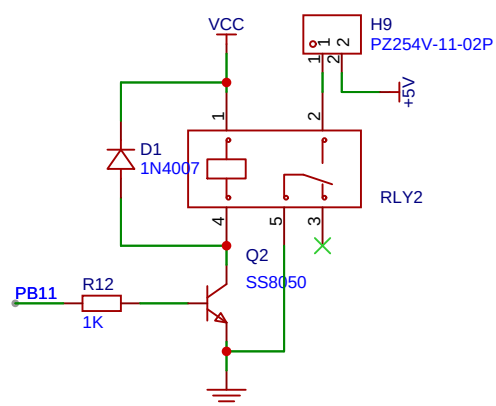
继电器电路
