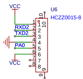
指纹立贴排针
