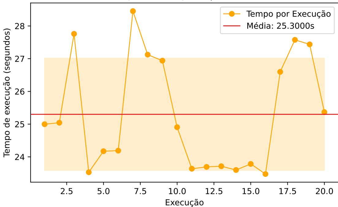
i06 - Desempenho Temporal | média=25.3000s
