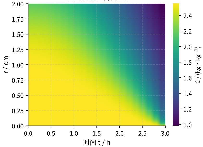
水分浓度场 C(r,t) 演化
