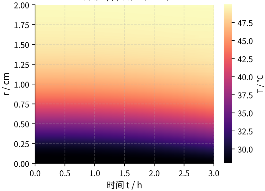
温度场 T(r,t) 演化 (0-3 h)
