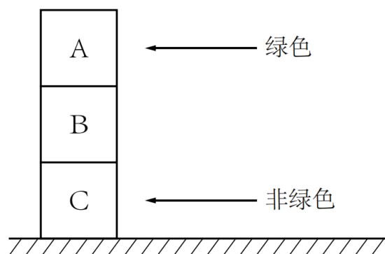
图 1: 方块世界
