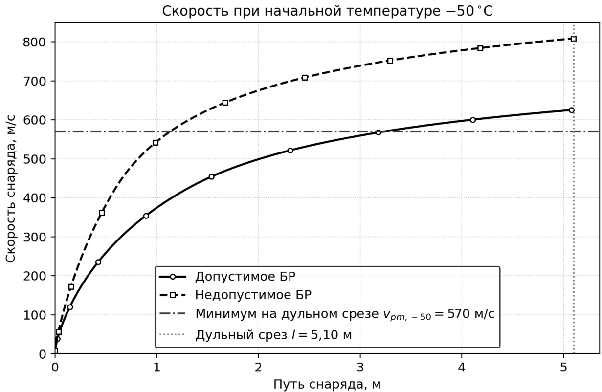
Рисунок 2 — Скорость снаряда при начальной температуре -50\text{ }^{\circ}\text{C}
