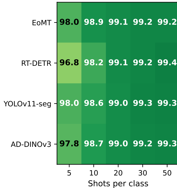
ViT-L/16
