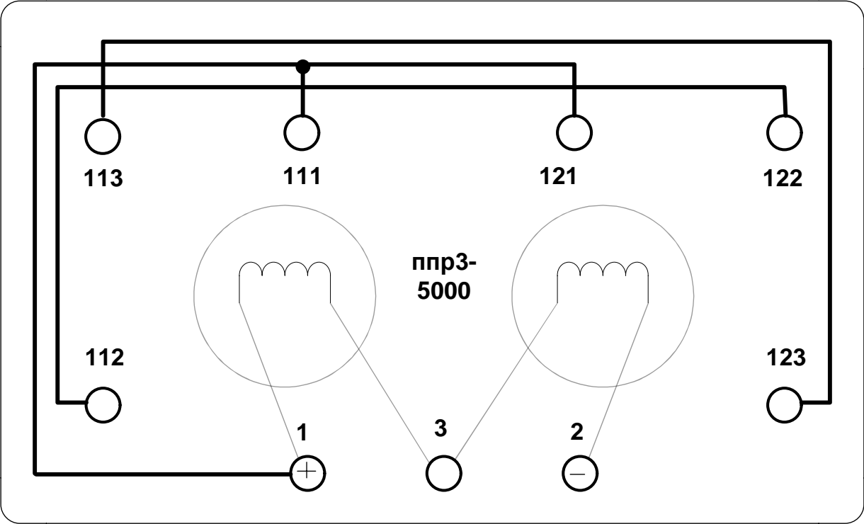
Схема перемичок ППРЗ-5000
