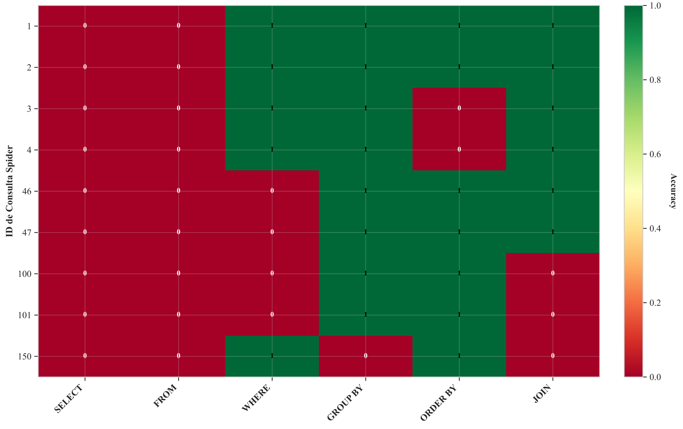
Precisión por Componente SQL en Spider Benchmark
