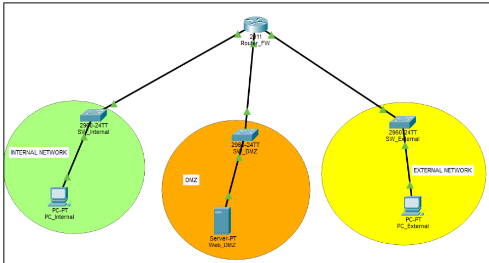
Figura 1. Topología general de la red en Packet Tracer
