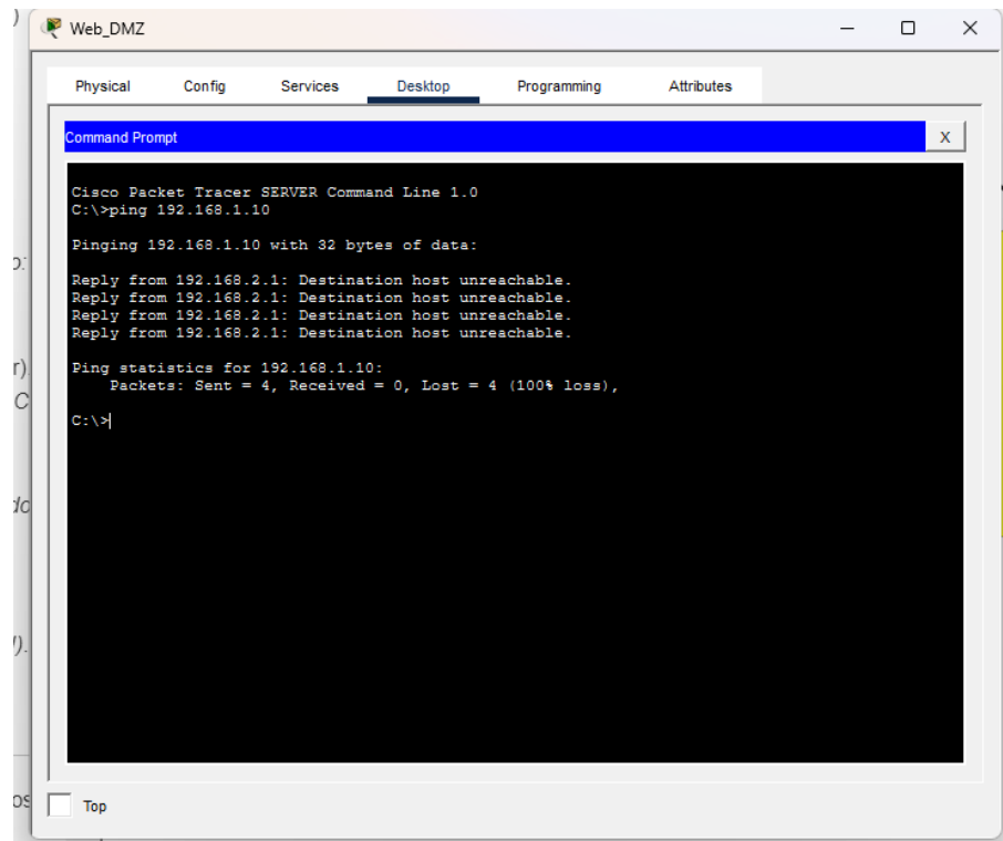
Figura 6. `ping` fallido desde `Server-PT Web_DMZ` a `PC_Internal` (bloqueado por ACL)
