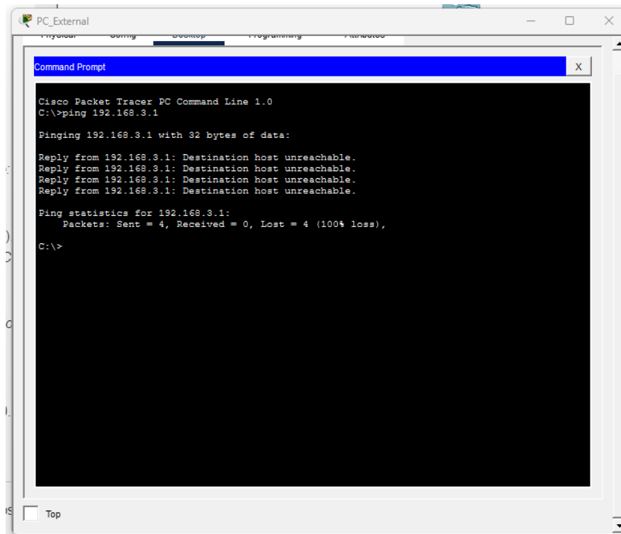
Figura 5. `ping` fallido desde `PC_External` a 192.168.3.1 (bloqueado por ACL)
