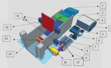
Gambar 3. Rancangan Alat
