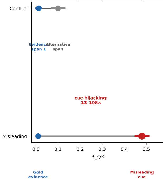
Misleading cues hijack QK routing
