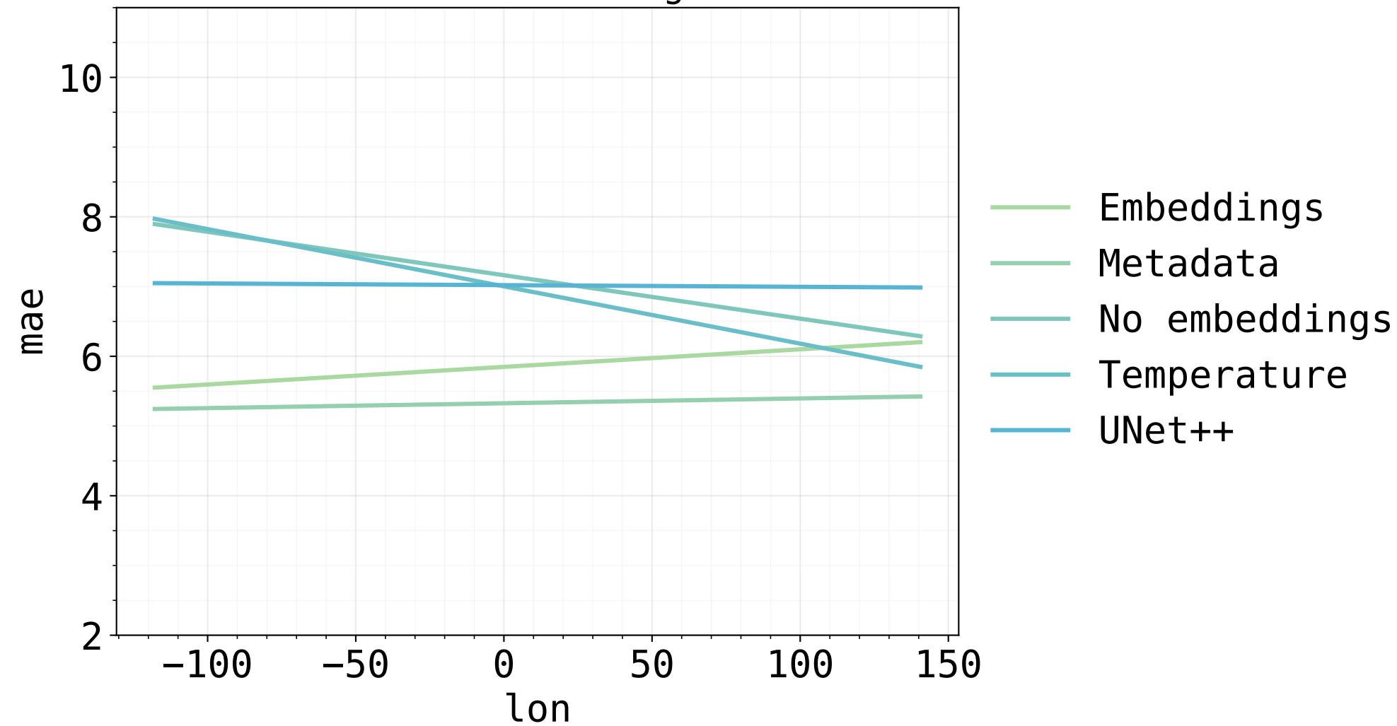
Trend: MAE vs Longitude
