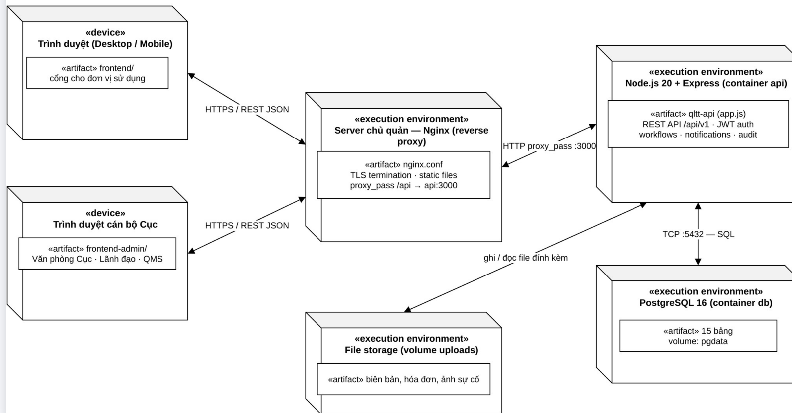
Sơ đồ triển khai — kiến trúc 3 lớp (Docker Compose)
