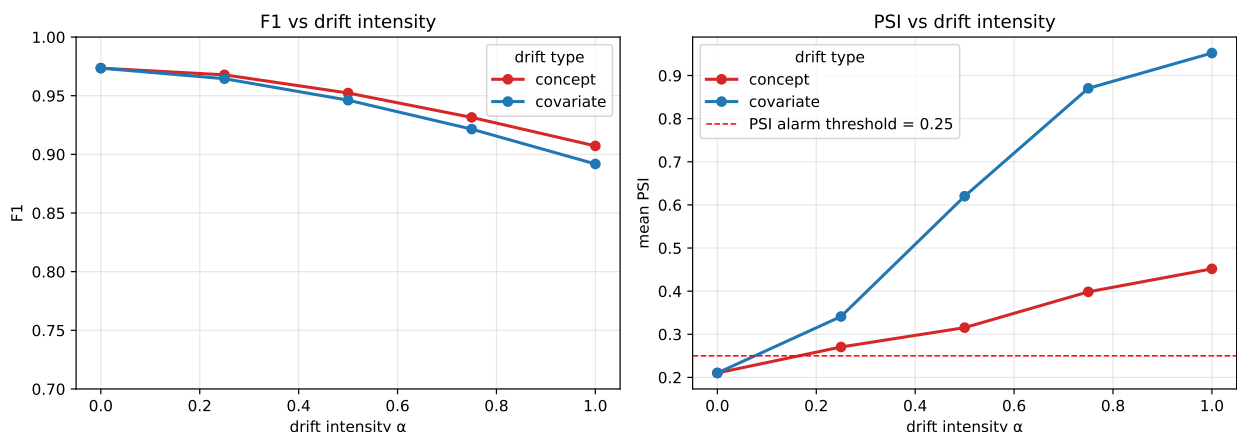
Рисунок 4.5 — Эксперимент E5: F1 и PSI vs интенсивность дрейфа для covariate и concept дрейфа; красная пунктирная линия в правой панели — порог \text{drift\_alarm} = 0,25
