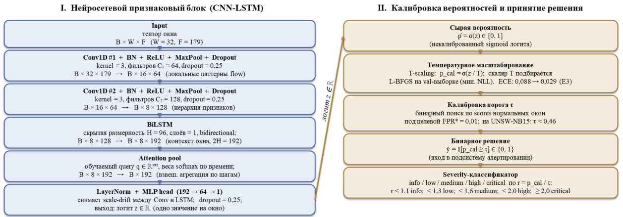
Рисунок 2.2 — Двухдорожечная блочная диаграмма детектора CNN-LSTM: дорожка I — извлечение признаков нейросетью; дорожка II — калибровка вероятностей и принятие решения
