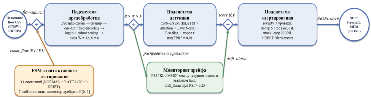
Рисунок 2.1 — Общая архитектура методики обнаружения: BPMN-схема потоков данных с параллельными ветвями мониторинга дрейфа и активного тестирования
