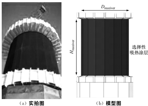
图7 圆柱形外露式吸热器结构图
